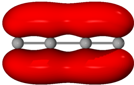
丁二烯 \pi_4^4
