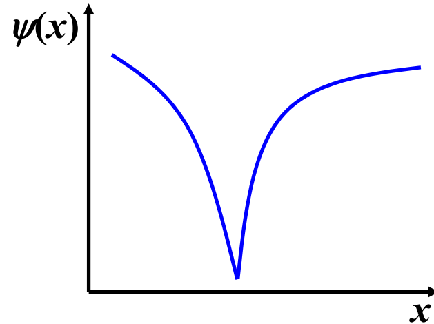
函数一级微商不连续
