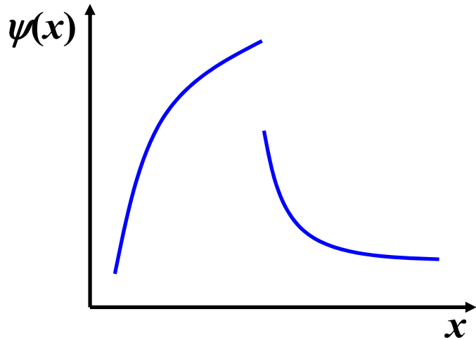
函数不连续
